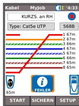
Abb. 31 Remote Kurzschlüsse
