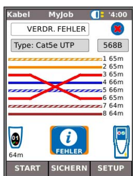
Abb. 28 Gekreuzte Paare
