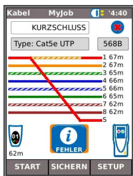
Abb. 30 Überbrückte Kurzschlüsse
